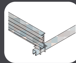
GRAPA PARA ANCLAJE DE CANAL ESTRUCTURAL A VIGA
