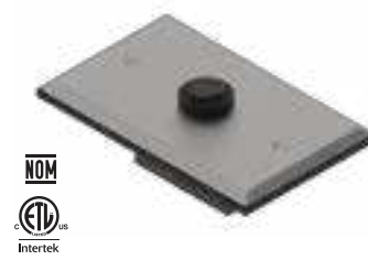
14 Placa metálica con fotocelda 120V 50-60Hz 4.2A 500W, tungsteno y 7.1A 850VA, balastro
