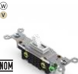
NOM 126 Pulsante para timbre 6A 125V~ 1P - Superficial
