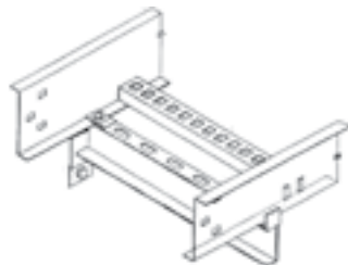
Ménsula montaje en pared - MP
